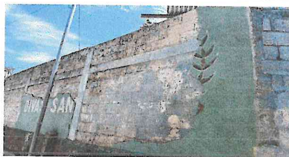
Foto 2: REPARACION DE MURO PERIMETRAL DE BLOCK, REFUERZO DE COLUMNAS, SOLERAS INTERMEDIAS
